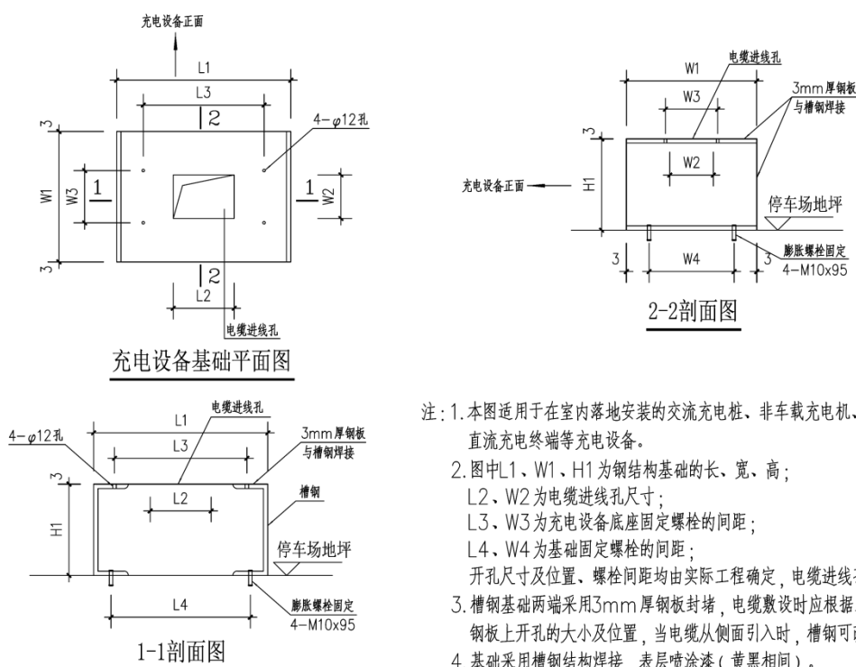
充电设备室内落地安装图示
