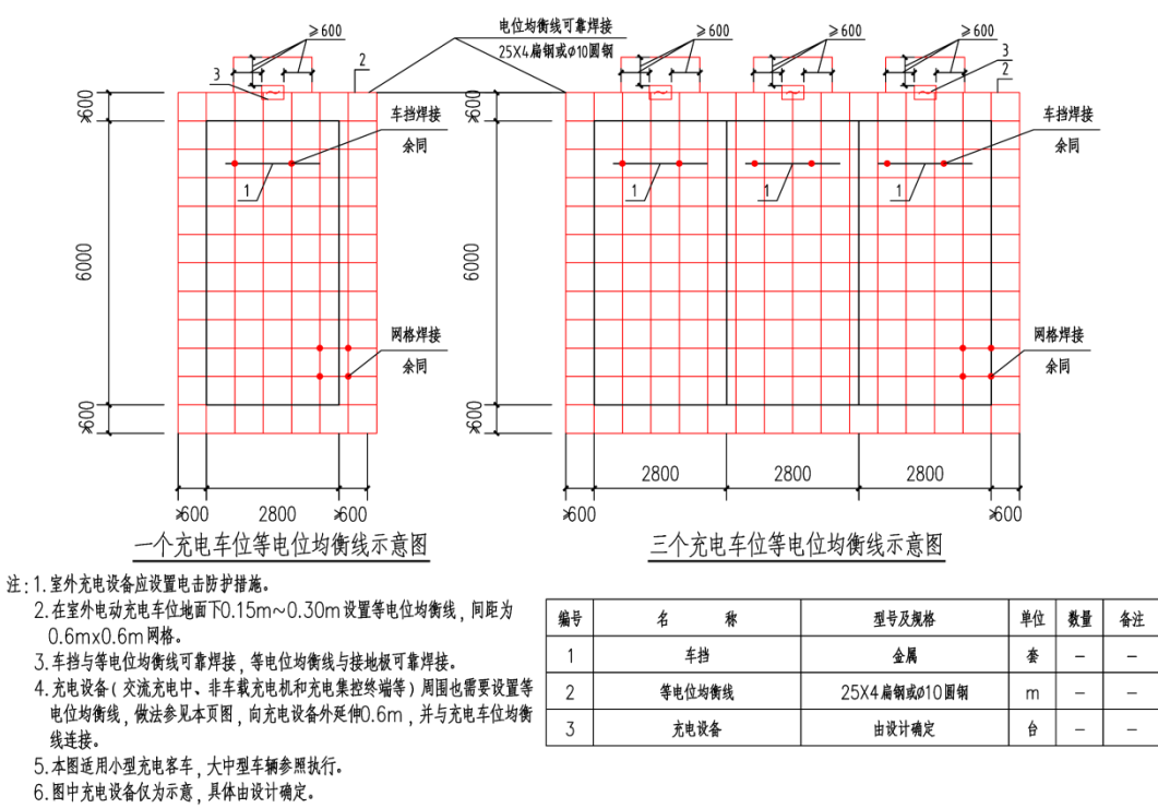
充电车位等电位均衡线示意图
