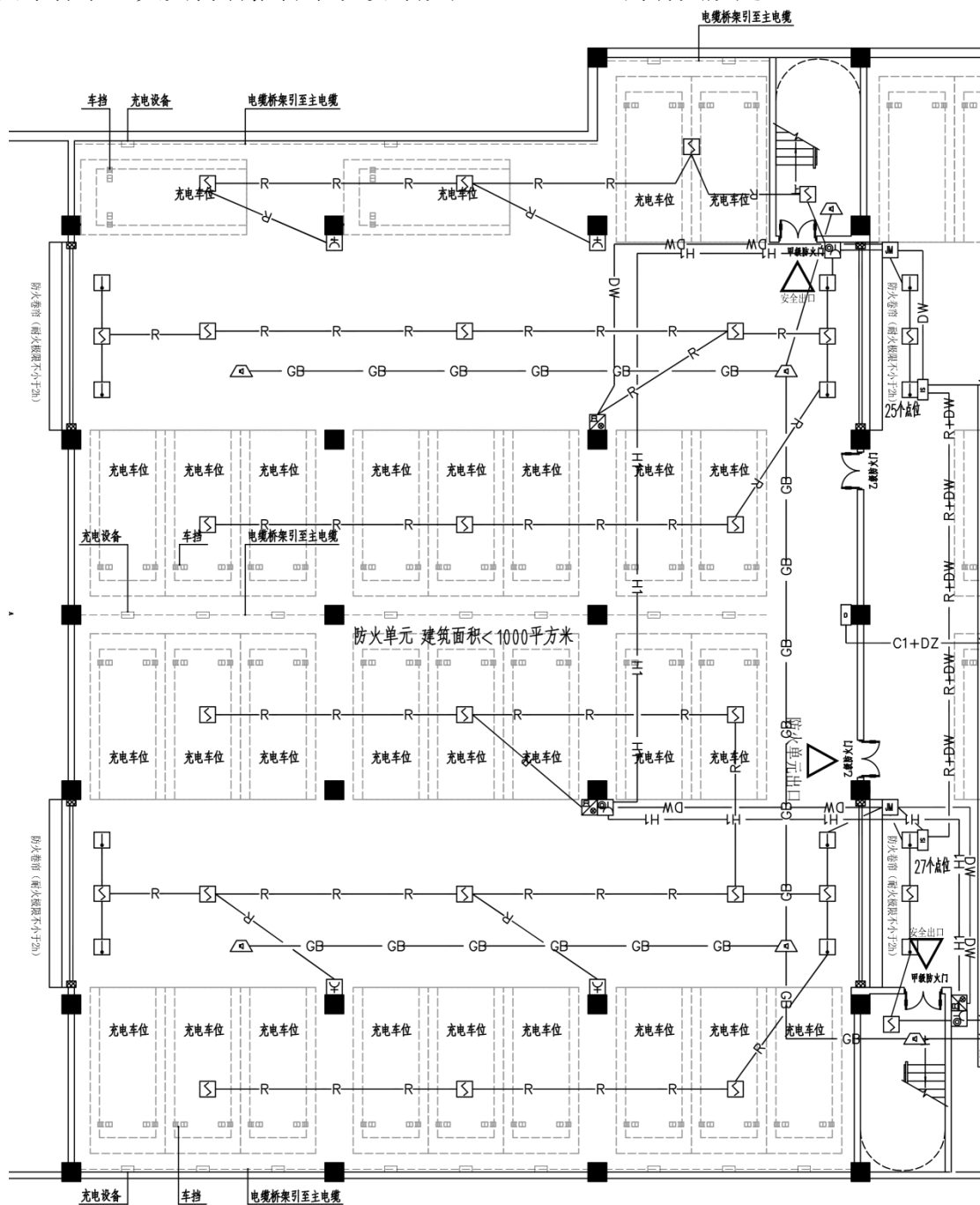
地下车库火灾自动报警布置示意图
