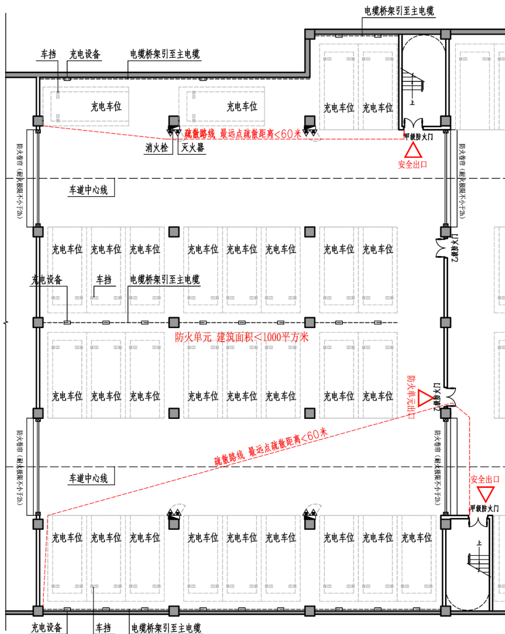
防火疏散示意图
