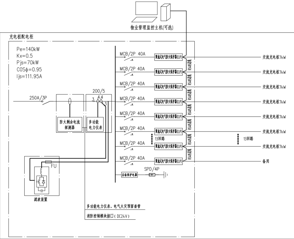
交流充电桩配电系统图
