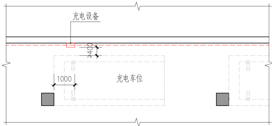
平行式停车充电设备与充电车位之间的距离示意
