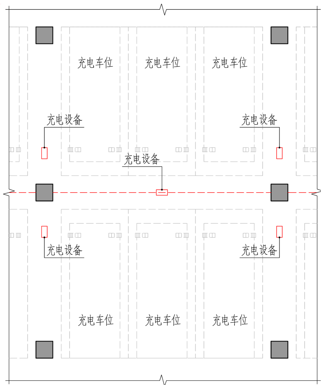
垂直式停车充电设备布置示意图
