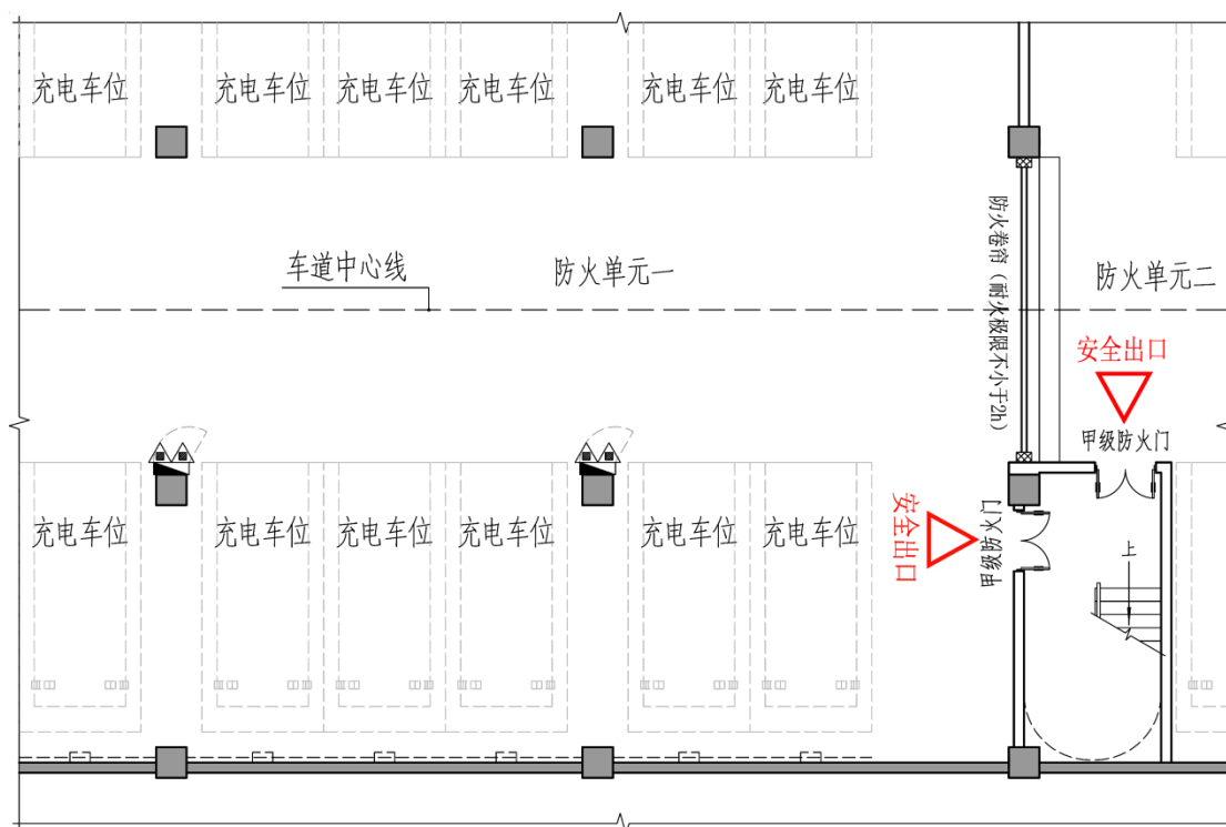
防火单元间疏散楼梯共用示意图
