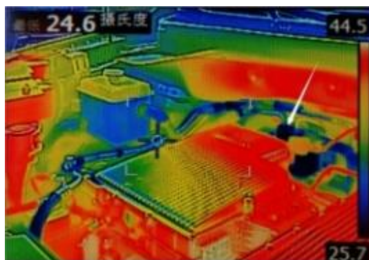
图 2 比亚迪 e1 电池热成像图
