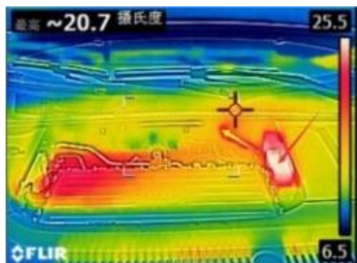
图 1 长城欧拉 R1 电池热成像图
