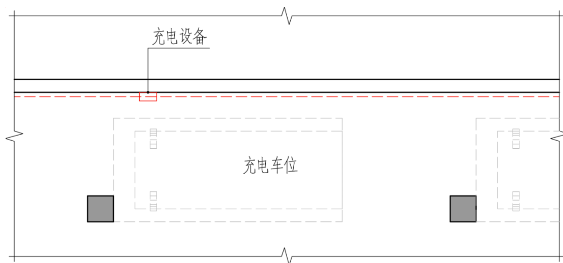
平行式停车充电设备布置示意图
