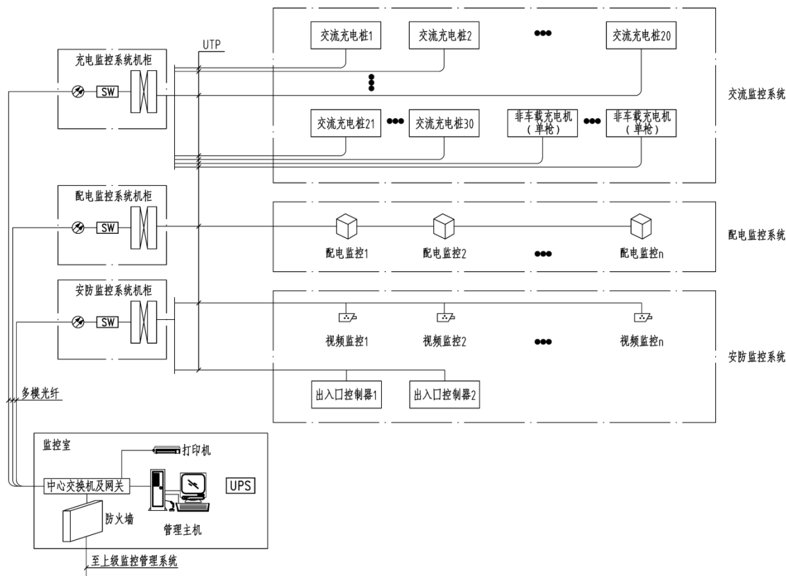
充电设施监控及管理系统示意图
