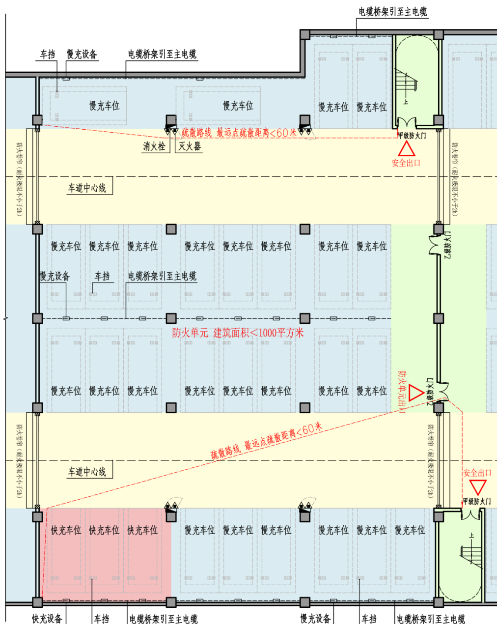
地下车库充电区布置示意图
