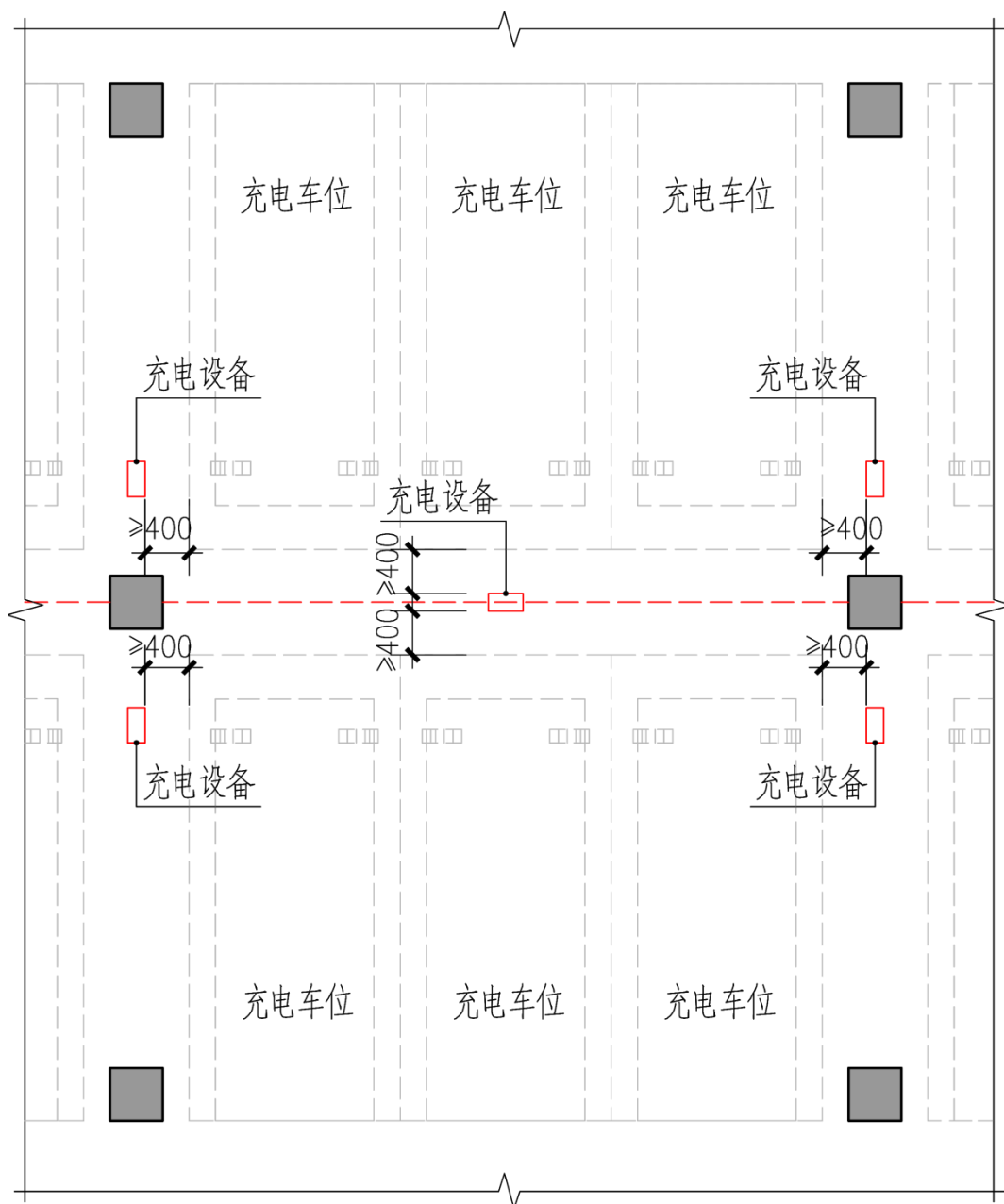
垂直式停车充电设备与充电车位之间的距离示意
