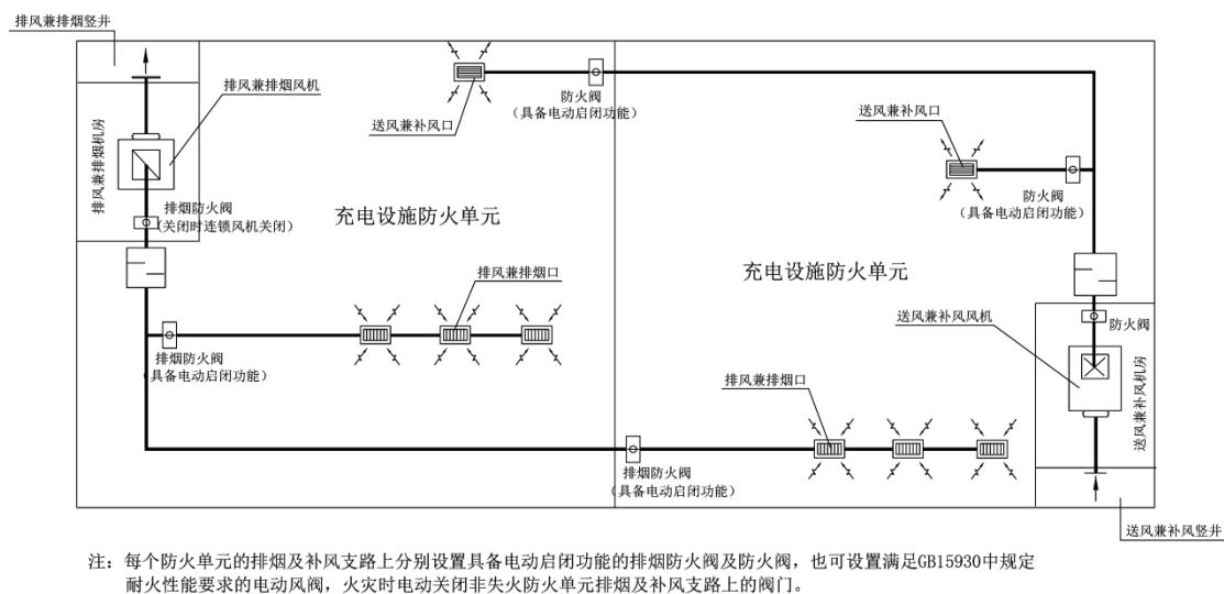
防火单元排烟、补风系统示意图
